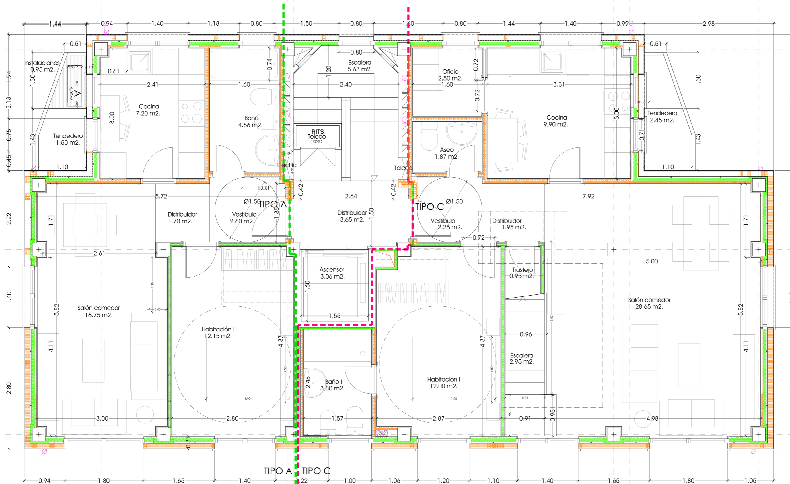
PLANTA CUARTA
