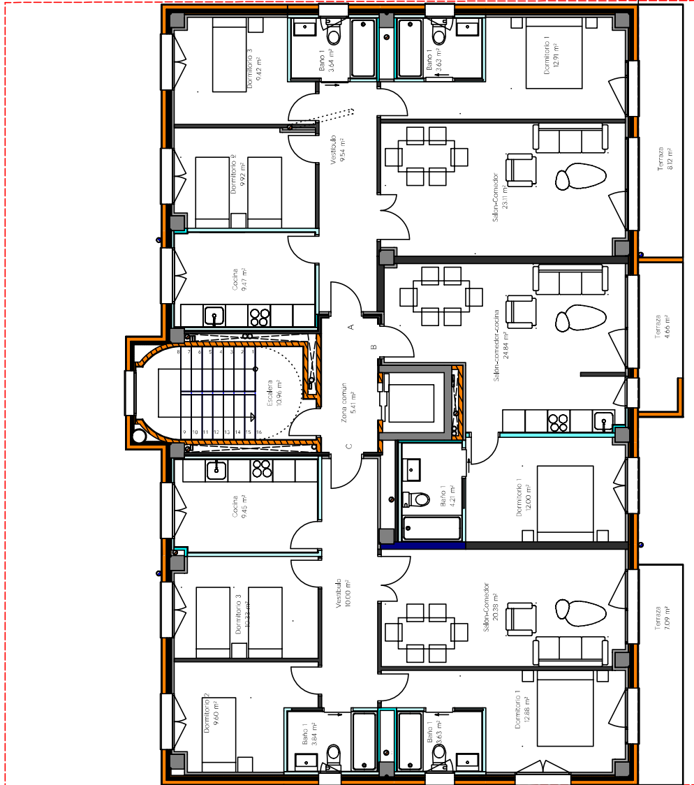
PLANTA 2
